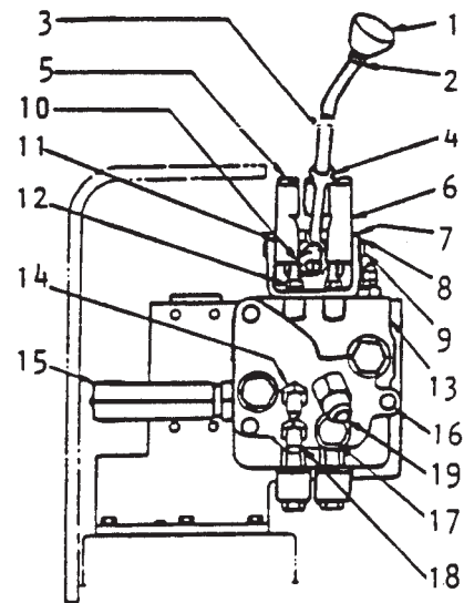
VÁLVULA-2 ÊMBOLOS
