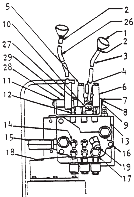
VÁLVULA-3 ÊMBOLOS
