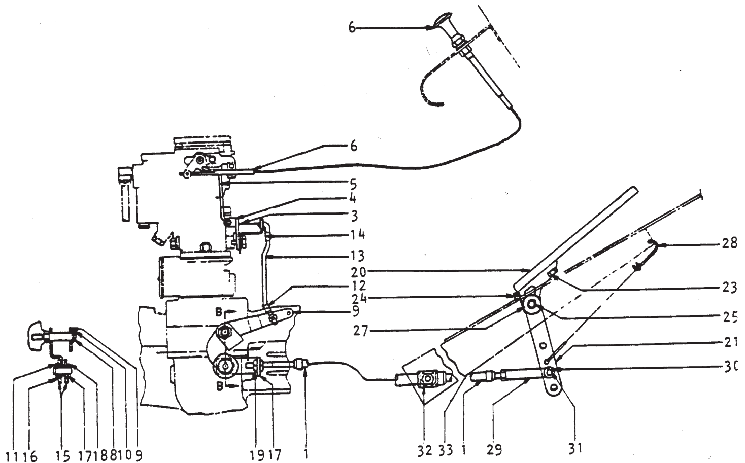
VISTA B
