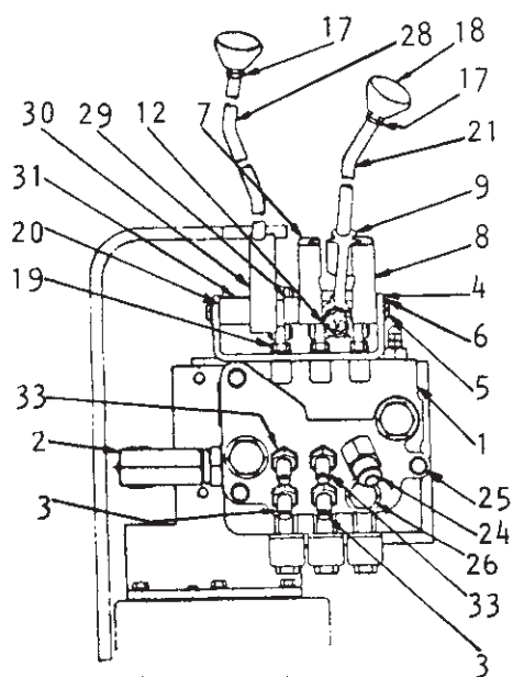
VÁLVULA 3 ÊBOLOS
