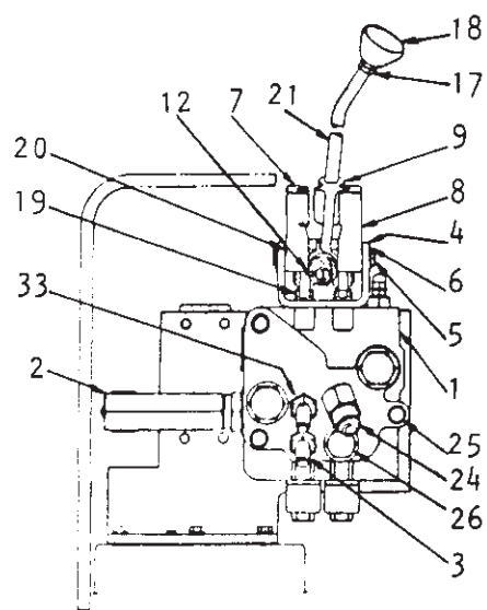
VÁLVULA 2 ÊBOLOS
