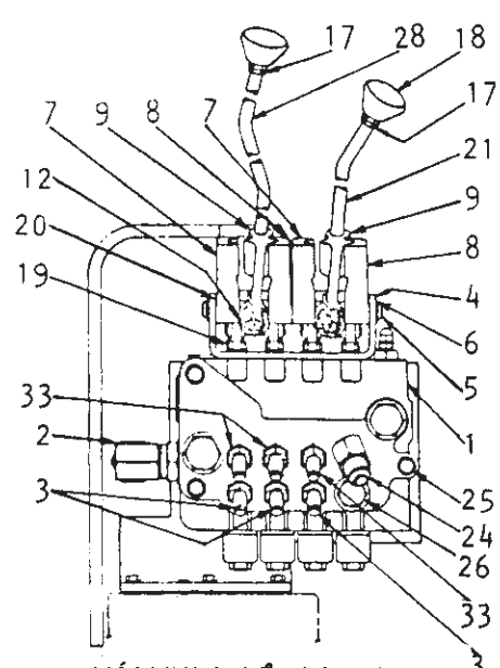
VÁLVULA 4 ÊBOLOS
