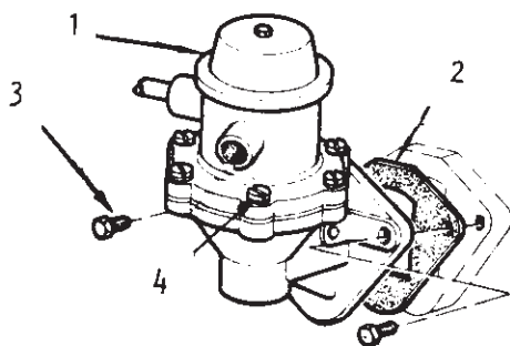
BOMBA "BROSOL"
