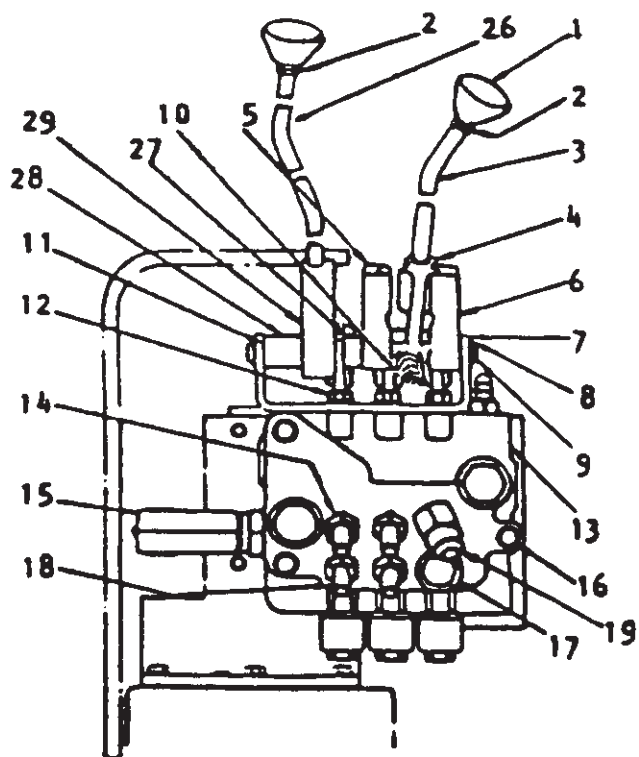
3 ÊMBOLOS
