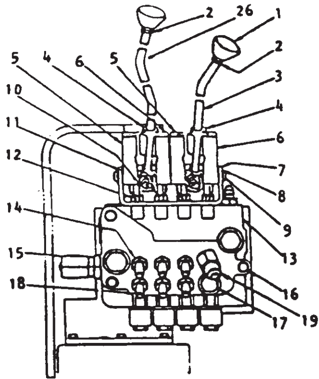
4 ÊMBOLOS
