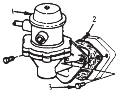
BOMBA "BROSOL"
