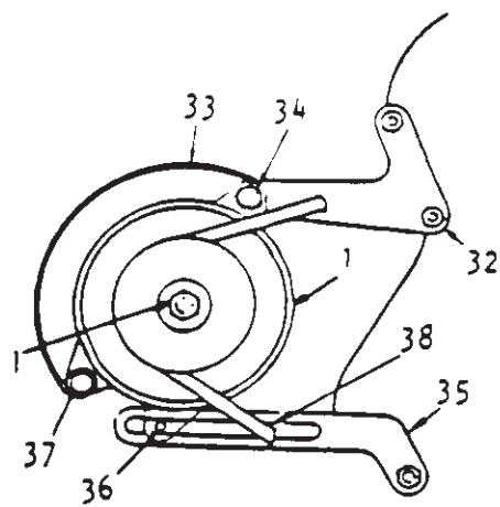
FIXAÇÃO DO ALTERNADOR
