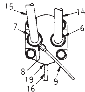
VISTA B
