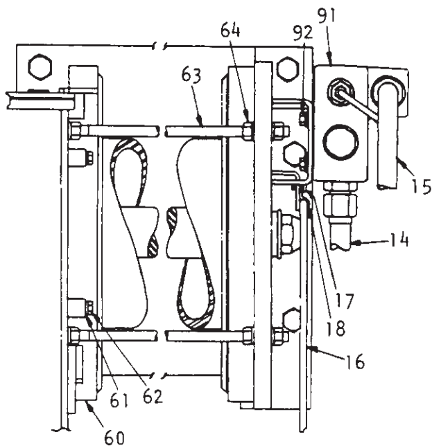
VISTA C
