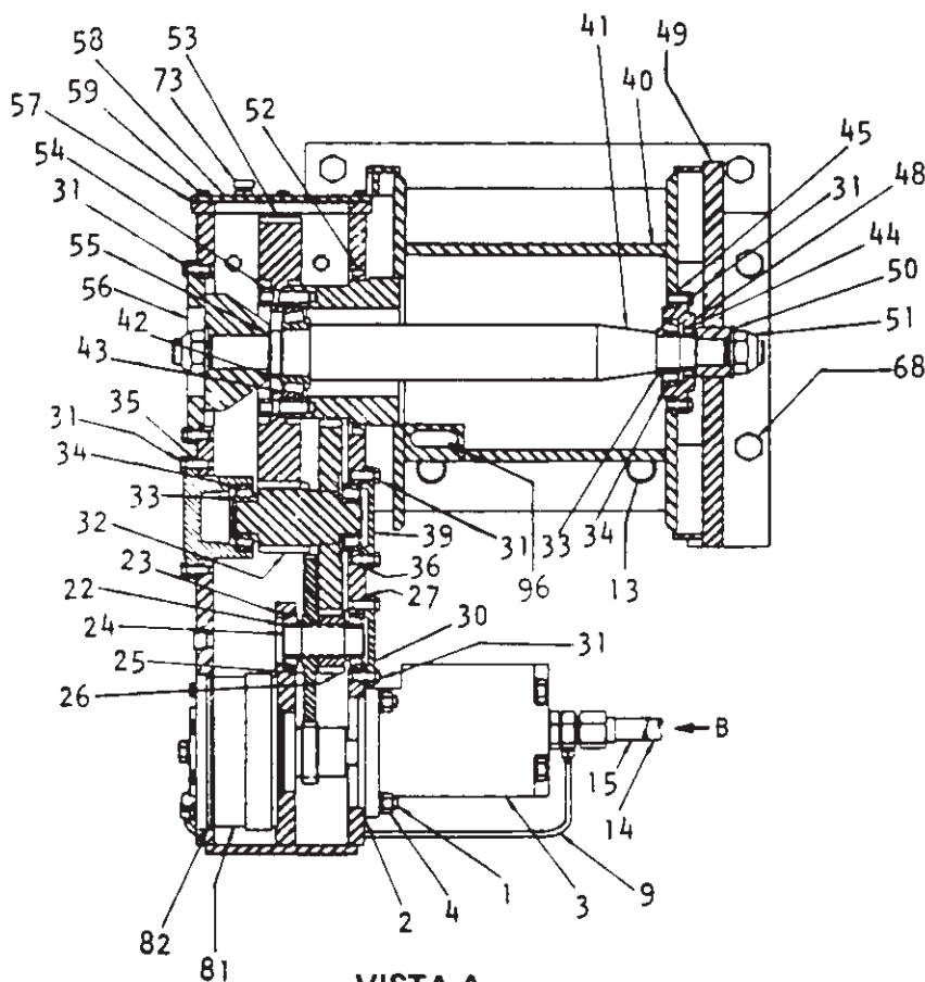
VISTA A
