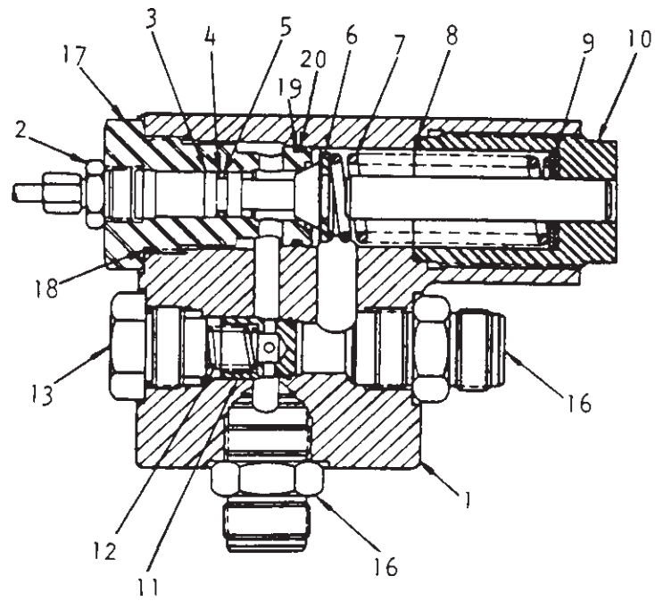
VISTA A
